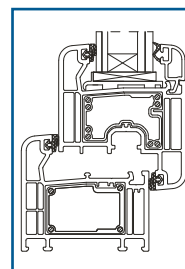
Nodo ANTA - TELAIO "L" telaio standard rinforzo termico
