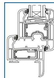
Nodo ANTA - TELAIO "Z" telaio restauro 27mm rinforzo termico
