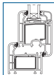
Nodo ANTA Mag. - TELAIO "L" telaio standard
