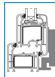
Nodo ANTA Mag. - TELAIO "L" particolare binario
